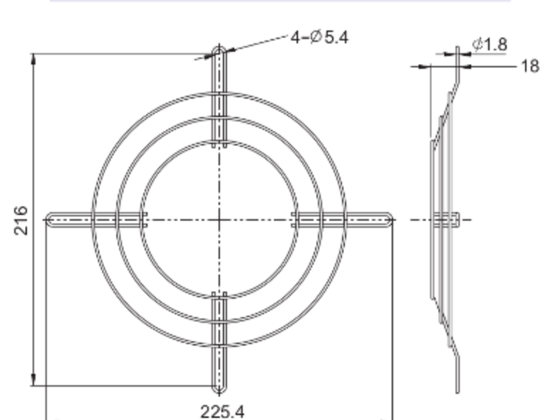
FG-18B For 176mm Fan
