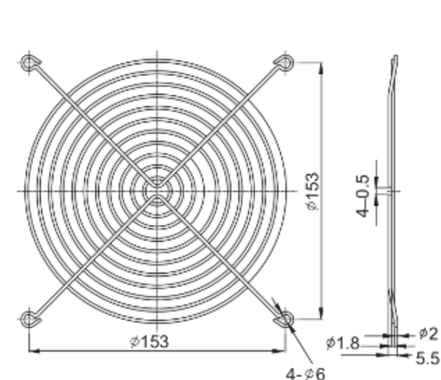
FG-18A For 176mm Fan
