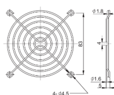
FG-09 For 92mm Fan
