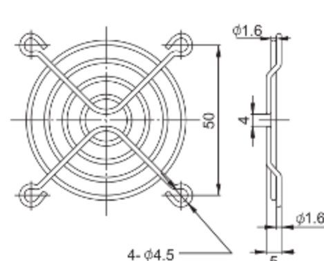
FG-06 For 60mm Fan
