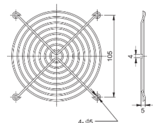
FG-12 For 120mm Fan
