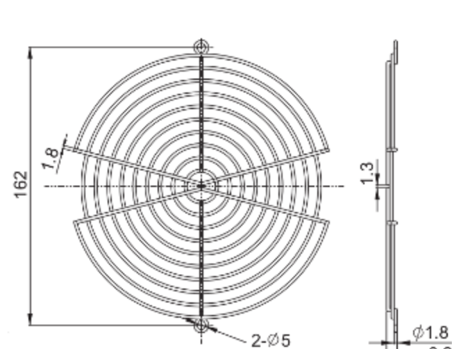
FG-17B For 172mm Fan
