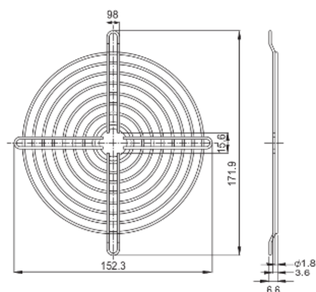
FG-18B For 176mm Fan
